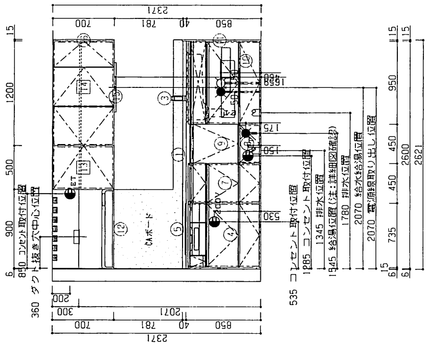
展開図A
